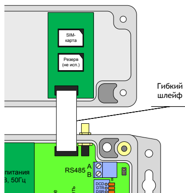
Рисунок 3. Разъем установки SIM-карты контроллера LitePro
