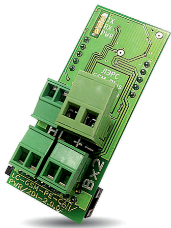
Платы расширения ЛЭРС GSM Plus устанавливаются в гнездо внутри корпуса контроллера.
