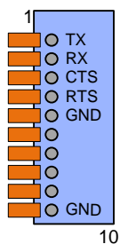
Рисунок 15. Разъем подключения RS-232 порта платы расширения
