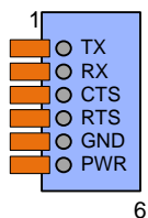
Рисунок 17. Разъем подключения RS-232 порта платы расширения
