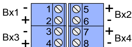
Рисунок 19. Разъем дискретных входов платы расширения
