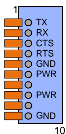
Рисунок 16. Разъем подключения RS-232 порта платы расширения
