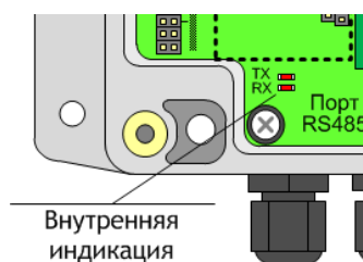
Рисунок 6. Внутренняя индикация
